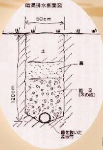
暗渠排水構造図
